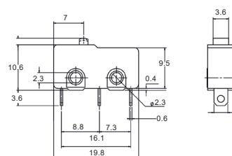
Button actuator
