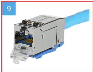
Fertig konfektioniertes Modul. A fully assembled module.
