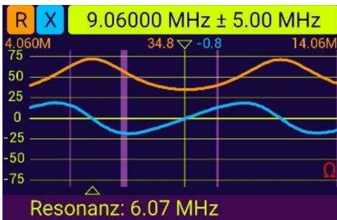
Beispiel 1: 50-Ohm-Kabel
